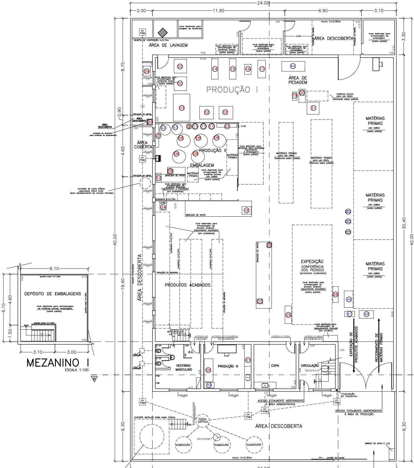
TÉRREO ESCALA 1:100
