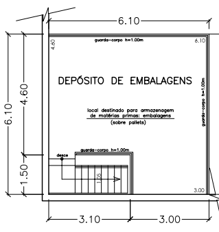
MEZANINO I ESCALA 1:100
