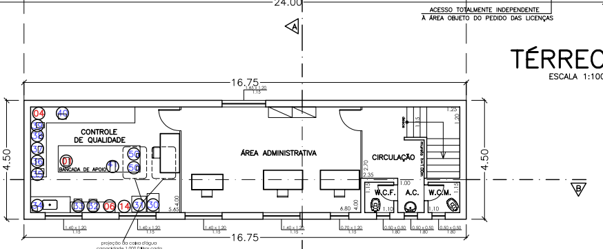
MEZANINO II ESCALA 1:100
